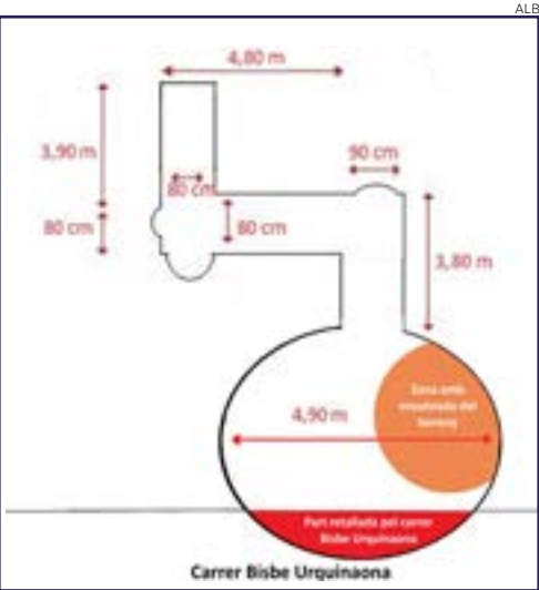
A l’esquerra, plànol actual de la fresquera del Mas de la Goma. A sobre d’aquestes línies, esquema de la fresquera de Can Rosés (Gavà)
