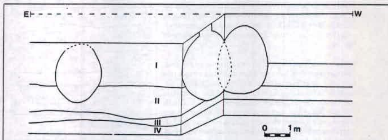
Fig. 2. Reconstrucció ideal del conjunt de les sitges 1 i 2 en relació al sediment quaternari.
