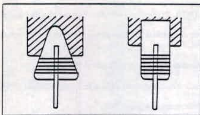
Fig. 6. Reconstrucció experimental de dos tipus de suport en fusta aptes per a subjectar la broca-perforador a l'extrem inferior del trepant.
