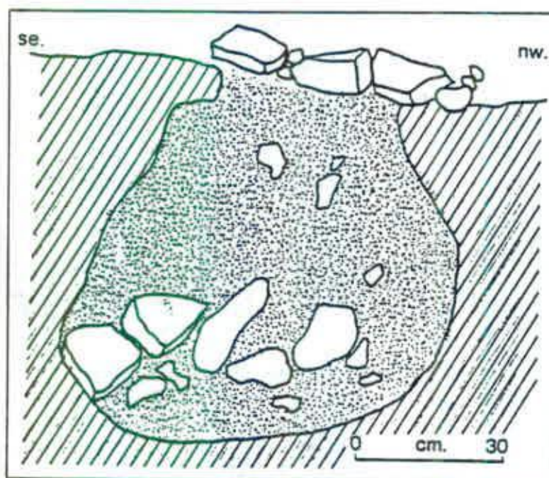
Fig. 3. Sitja 1. Secció transversal.
